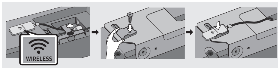
Viena stiprinājuma tips (WMN300SB, neietilpst komplektācijā)
