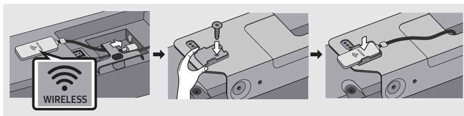
Ühe kinnitusega tüüp (WMN300SB, ei kuulu komplekti)
