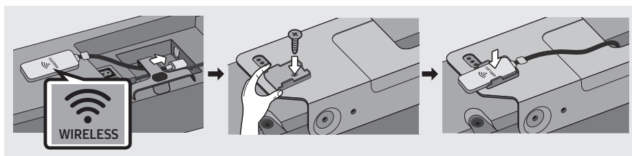
Vieno laikiklio tipas (WMN300SB, nepridedamas)
